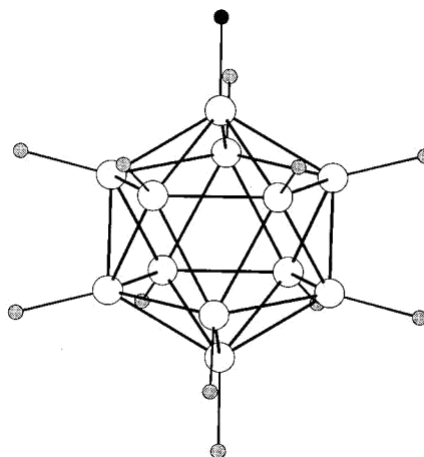
(d) closo - [B_{12}H_{12}]^{2-}
